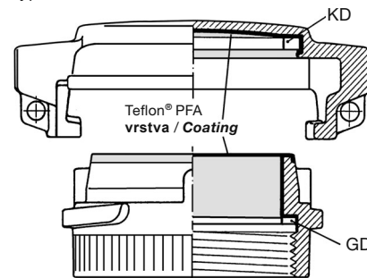
Typ VK ... SSE
