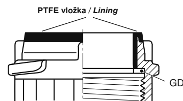
Typ VK ... SSE PTFE
