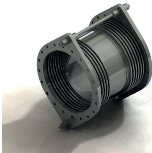
MFL Univerzálny kompenzátor s tiahľami a pevnými prírubami.
